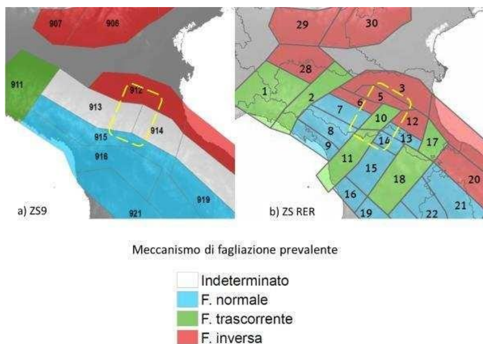
Figura 9 – a particolare della zonazione sismogenetica ZS9 (Meletti e Valensise, 2004); b) particolare della zonazione sismogenetica proposta dalla Regione Emilia-Romagna (Martelli et al., 2017b); il perimetro tratteggiato giallo indica l'area d'interesse.
