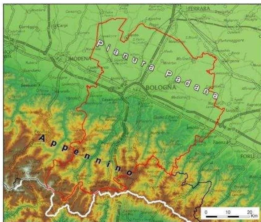
Figura 1 – Inquadramento geografico e morfologico dell'area d'interesse; in rosso il confine della Città Metropolitana, in nero il confine regionale, in bianco lo spartiacque appenninico.
