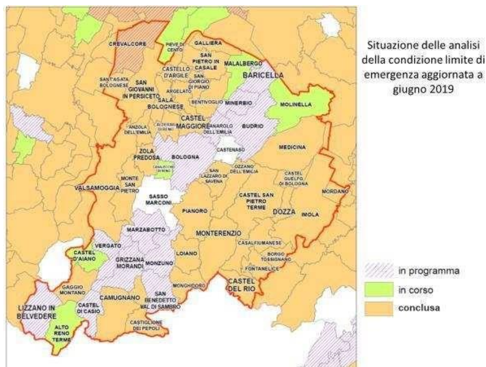
Figura 13 - Stato dell'arte delle analisi della condizione limite di emergenza; in rosso il perimetro della Città Metropolitana
