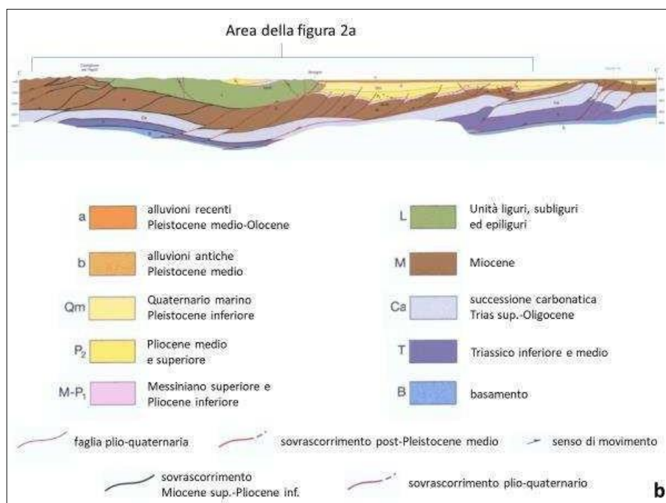
Figura 2 – a) mappa geologica e b) sezione geologica dell'area d'interesse. In figura 2a il perimetro nero indica i confini della Città Metropolitana, la linea blu è traccia della sezione di figura 2b.
