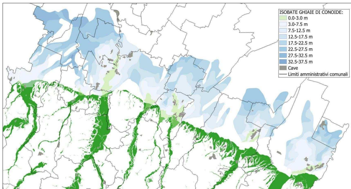
Figura 15 – Rielaborazione della profondità del tetto dei depositi grossolani di conoide rispetto alle quote di campagna.
