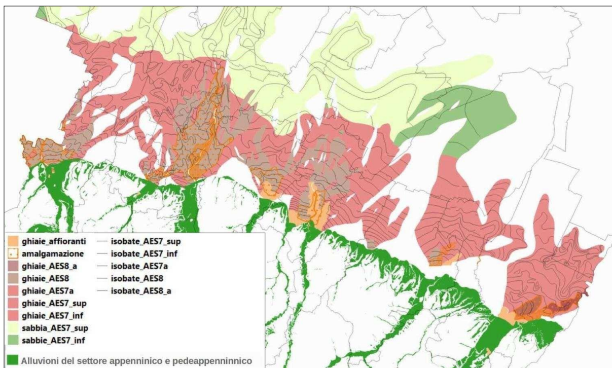
Figura 14 - Ricostruzione dei depositi grossolani di conoide nel territorio metropolitano di Bologna (fonte: Banca Dati SGSS RER).
