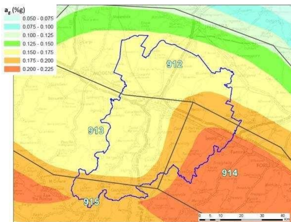
Figura 10 – Mappa di pericolosità sismica di base per l'Emilia-Romagna e zone limitrofe, TR= 475 anni (Gruppo di lavoro MPS, 2004); i colori indicano le classi di a_g , accelerazione di picco su suolo rigido e pianeggiante, espressa in percentuale dell'accelerazione di gravità g ; in blu il perimetro della Città Metropolitana, in nero i limiti delle zone sismogenetiche ZS9.
