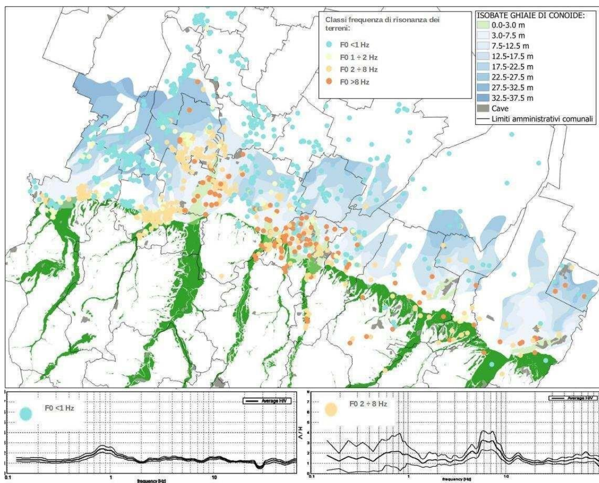
Figura 16 – Confronto tra limiti e profondità dei depositi grossolani di conoide e le misure dei microtremori sismici HVSR (prove eseguite per gli studi di MS comunali).
