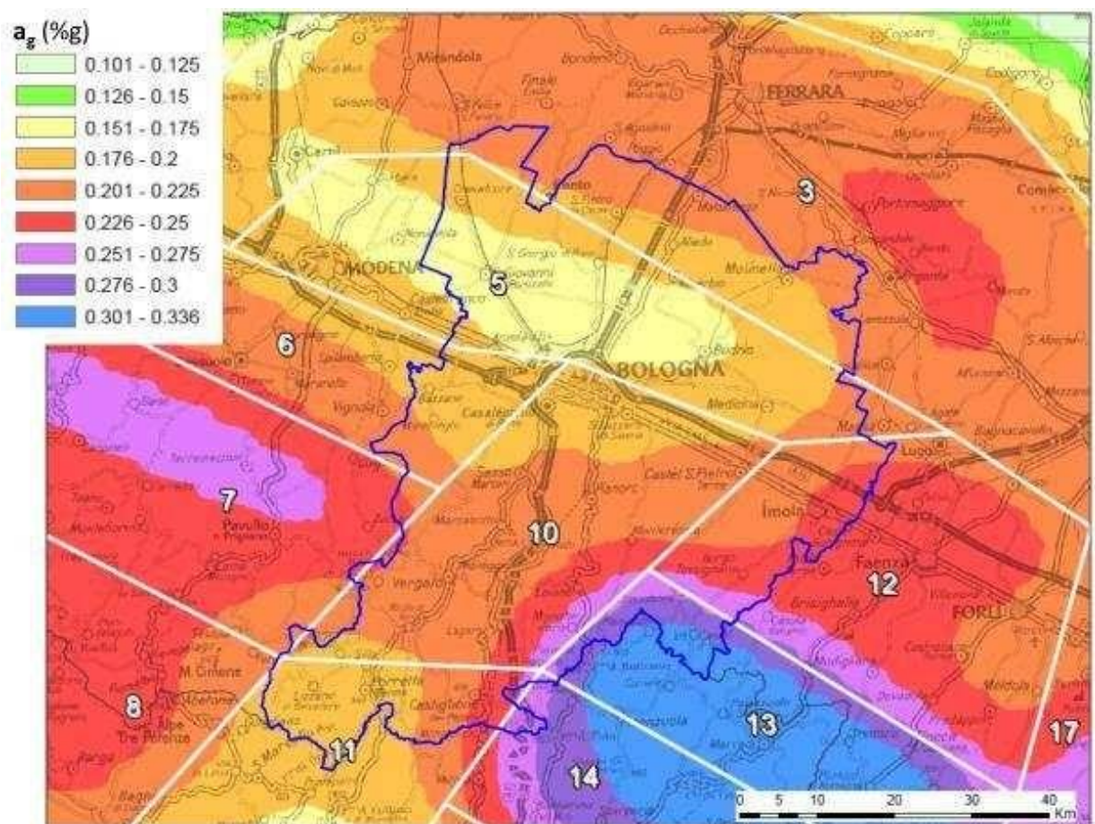
Figura 11 - Mappa di pericolosità sismica di base per l'Appennino settentrionale e zone limitrofe sulla base di un modello 3D delle sorgenti sismiche (Martelli et al., 2017b), TR=475 anni; i colori indicano le classi di a_g , accelerazione di picco su suolo rigido e pianeggiante, espressa in percentuale dell'accelerazione di gravità g ; in blu il perimetro della Città Metropolitana, in bianco i limiti delle zone sismogenetiche ZS RER.
