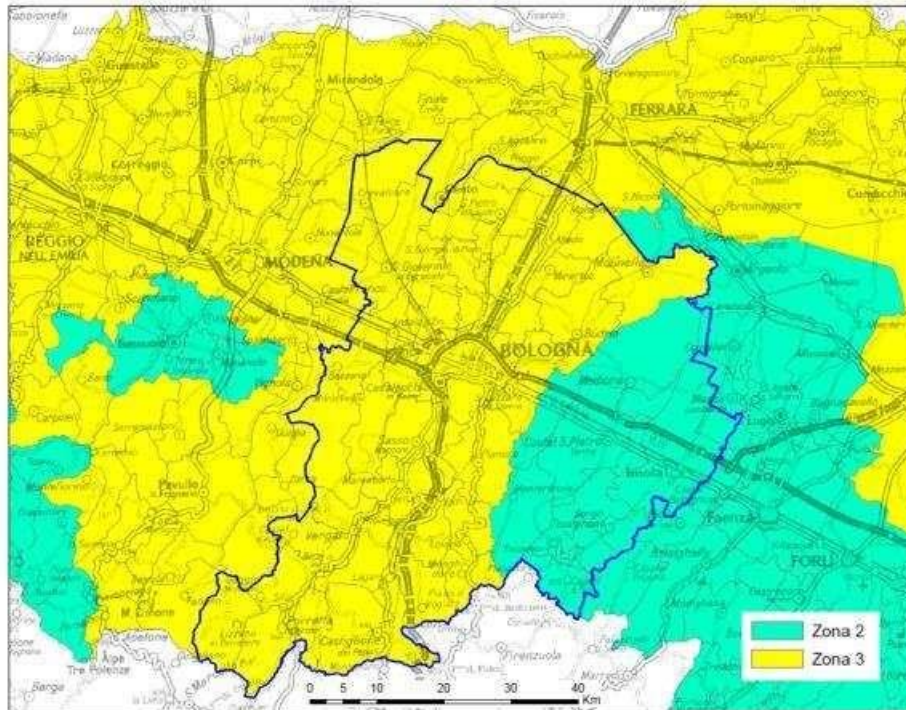
Figura 5 - Classificazione sismica della Città Metropolitana e aree limitrofe.
