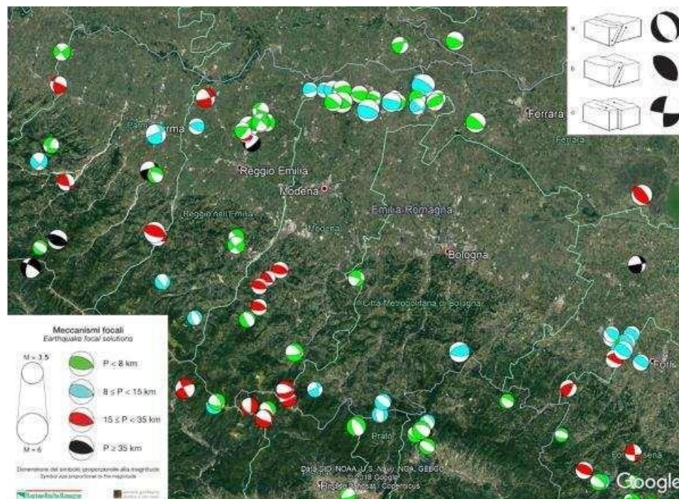
Figura 7 – Meccanismi focali del territorio bolognese e aree limitrofe (da Martelli et al., 2017a, e http://terremoti.ingv.it ). Simboli: i colori indicano le classi di profondità (v. legenda in basso a sinistra), le zone a campitura piena i quadranti in estensione (v. legenda in alto a destra: a) meccanismo distensivo, b) meccanismo compressivo, c) meccanismo trascorrente).
