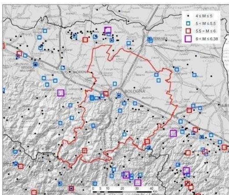
Figura 3 – Epicentri dei principali terremoti ( M_W \geq 4 ) a partire dall'anno 1000 (da Rovida et al., 2016); in rosso il perimetro della Città Metropolitana.
