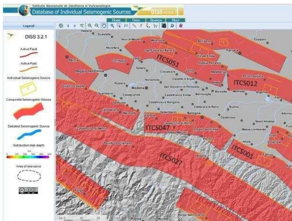
Figura 8 – Strutture sismogenetiche capaci di generare di forti terremoti ( MW \geq 5.5 ), da DISS 3.2.1 (DISS Working Group, 2018)
